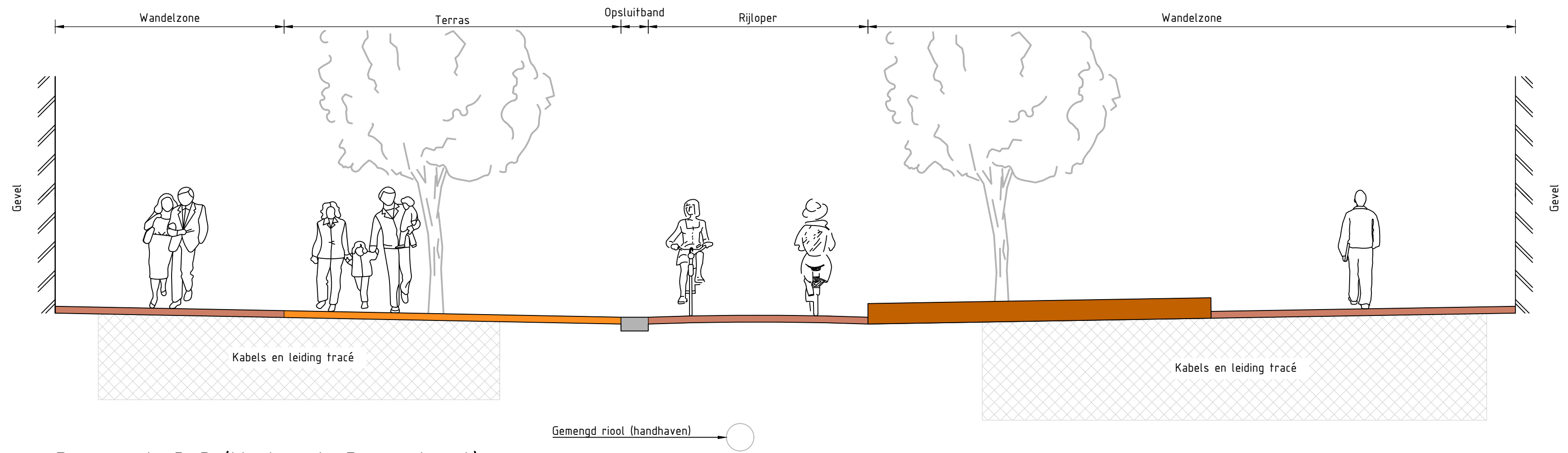
Doorsnede B-B (Verlengde Dorpsstraat) schaal 1:50
