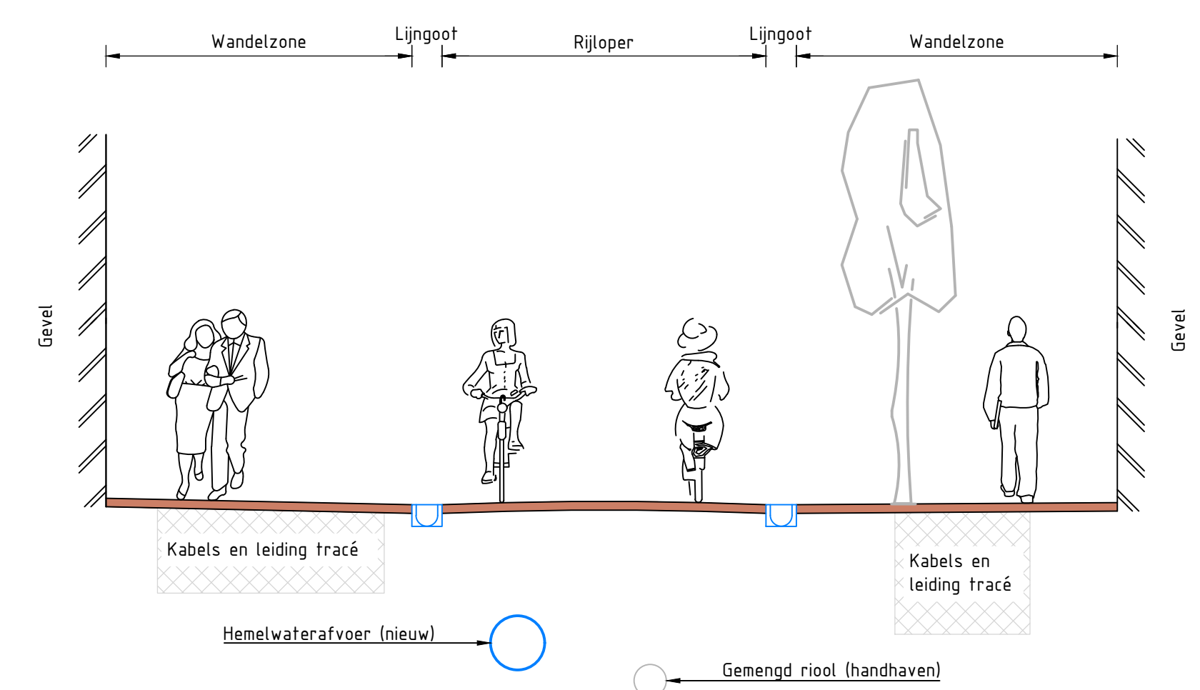
Doorsnede D-D (Kerkstraat) schaal 1:50
