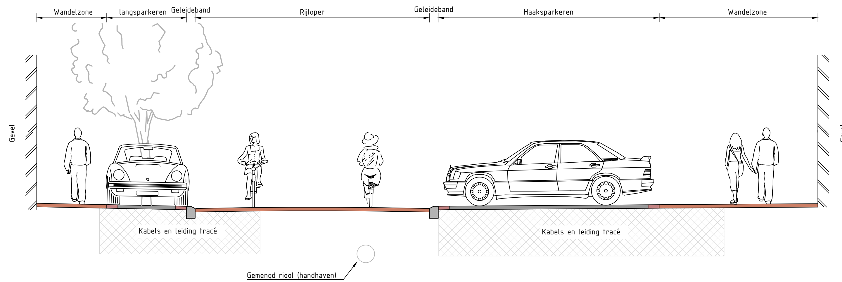
Doorsnede C-C (Verlengde Dorpsstraat) schaal 1:50
