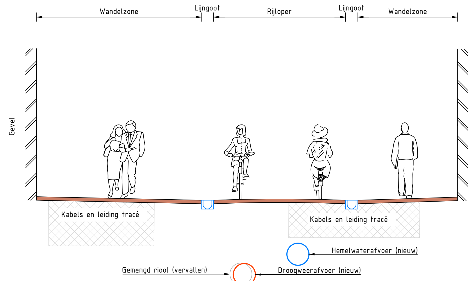
Doorsnede A-A (Dorpsstraat) schaal 1:50
