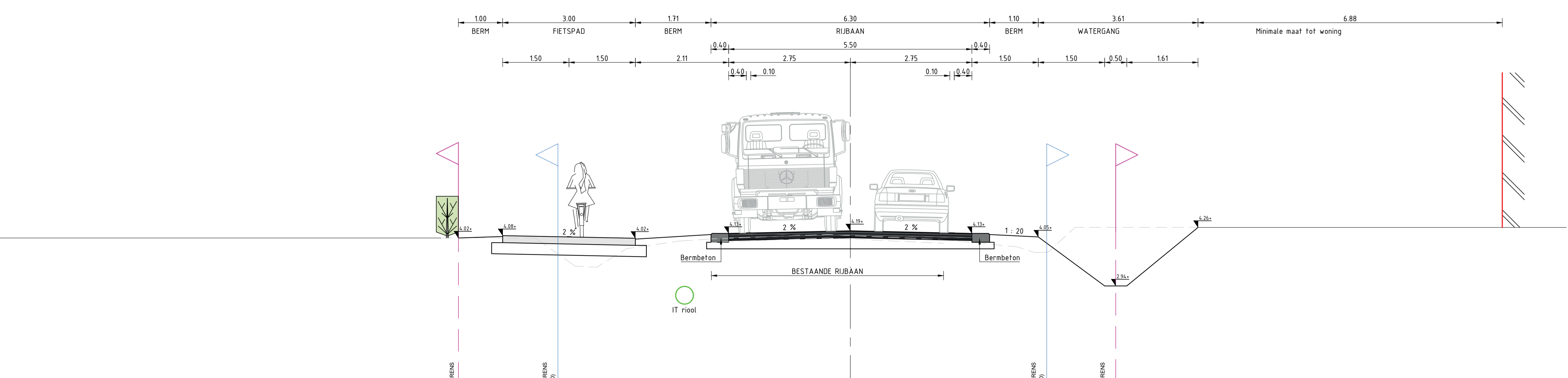
Profiel L-L 1:50
