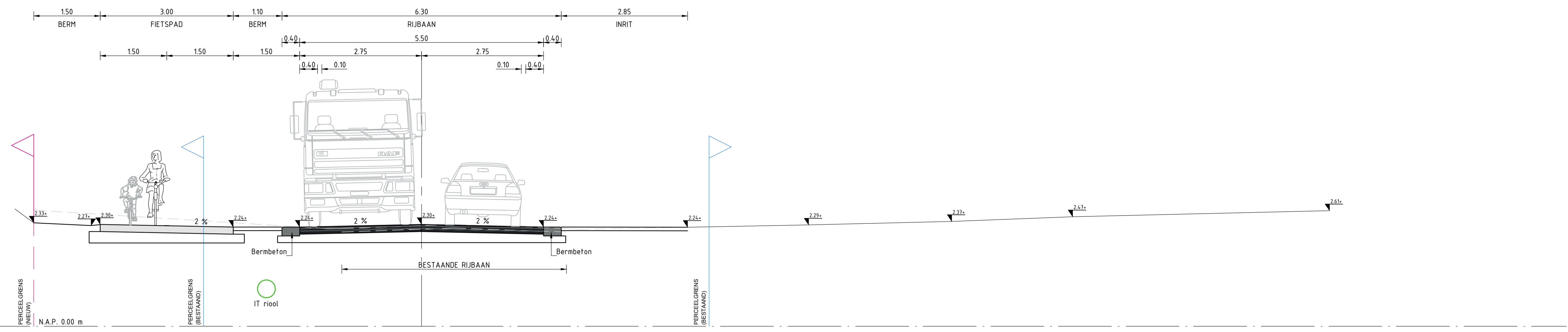
Profiel E-E 1 : 50
