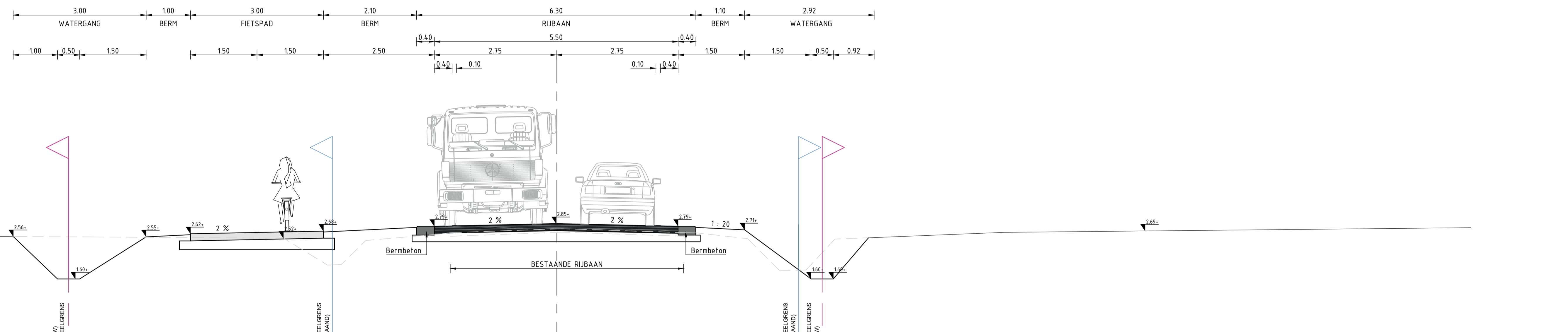
Profiel H-H 1 : 50
